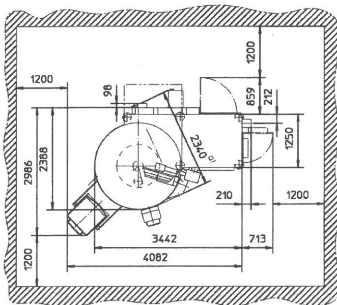
a) erforderliche Türweite bei demontiertem Bedienpult required door width in case of detached control panel
